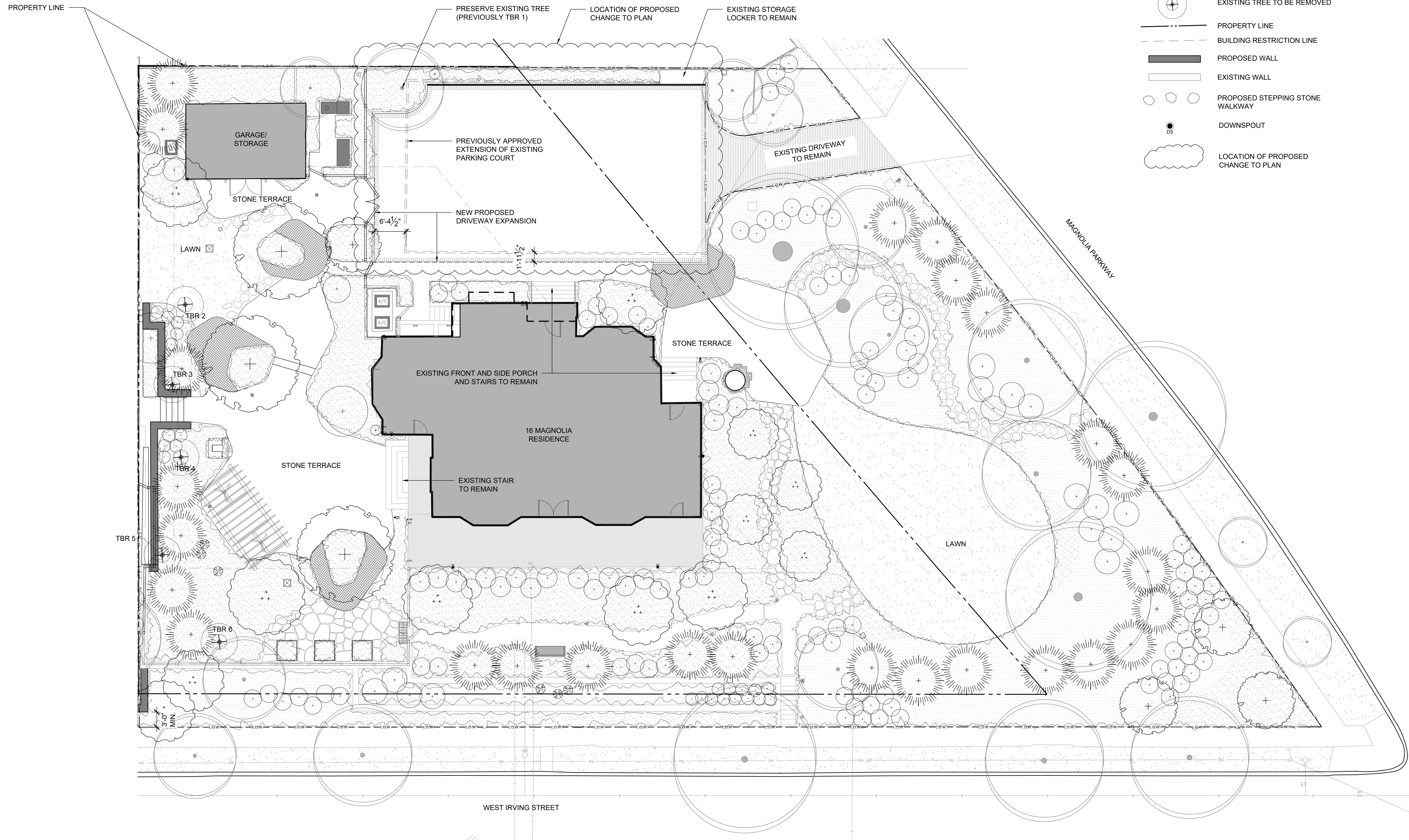
A 16 MAGNOLIA PKWY SITE PLAN
